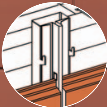
PROFIL SA ZATVORENIM SPOJEM NO: DWG 200-06, SPOJ 9 MM
