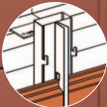
PROFIL SA OTVORENIM SPOJEM NO: DWG 200-13, SPOJ 9 MM
