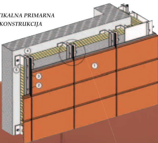
HORIZONTALNA PRIMARNA PODKONSTRUKCIJA
