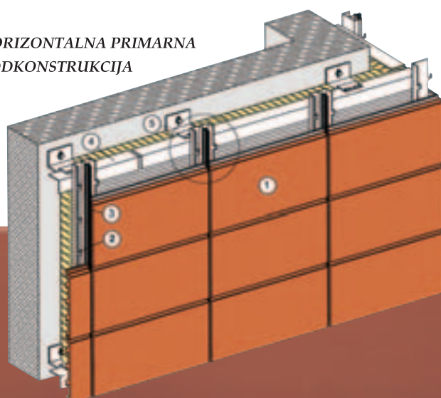
KLASIČNI SISTEM (CLS) NA HORIZONTALNOJ PRIMARNOJ PODKONSTRUKCIJI
